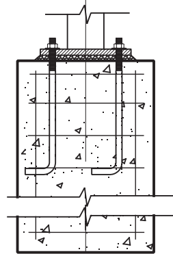
USING L-BOLTS
